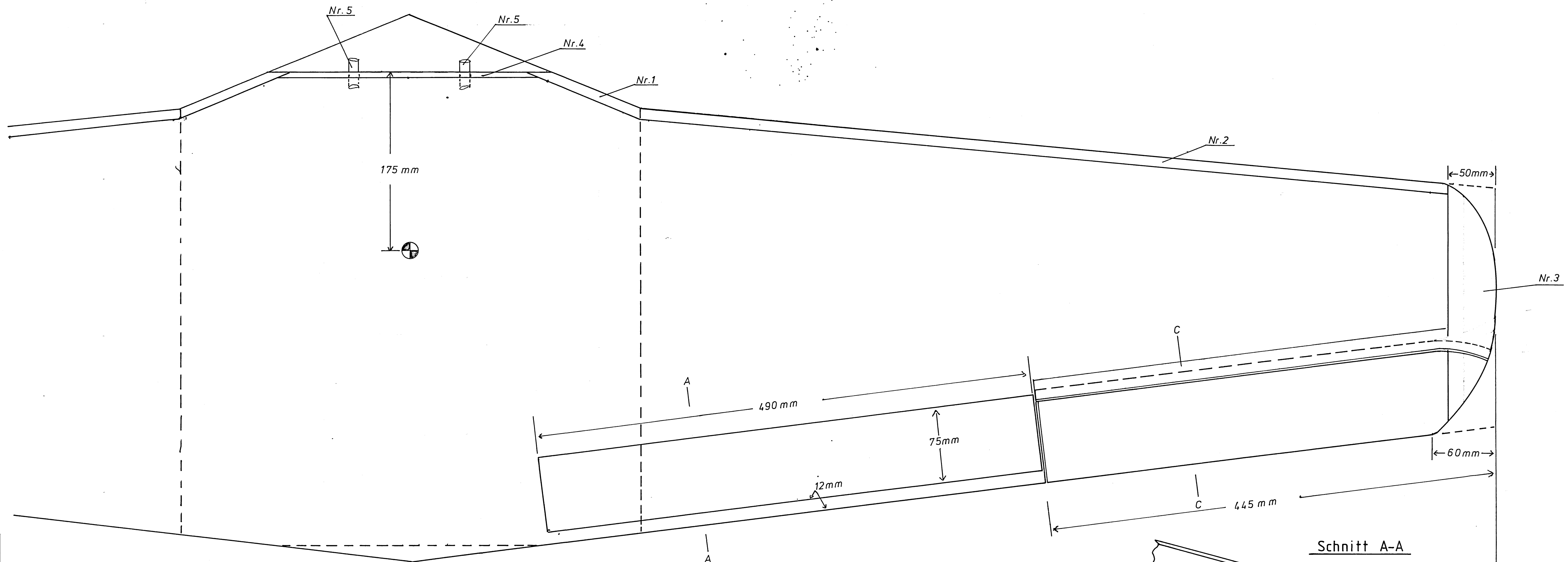
Landeklappen 1:1
