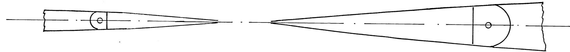
Seitenruder M 1:1
